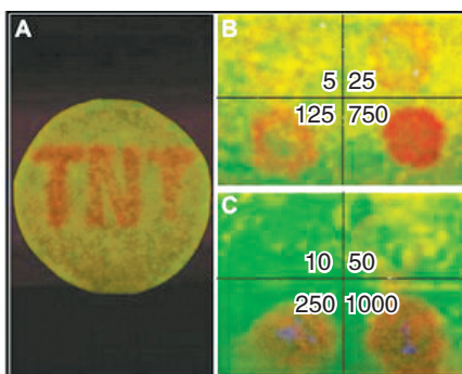
纸质传感器对不同表面梯恩梯含量变化的可视化显色效果
